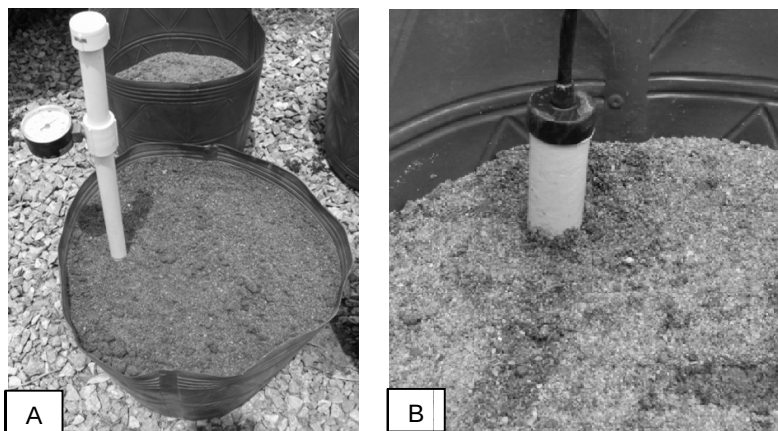
Figura 2 – Detalhe do tensiômetro (A) e do sensor Irrigas instalados nos vasos para monitoramento da tensão de água no substrato.
