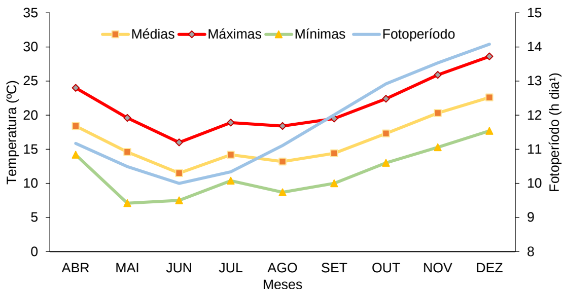
Figura 1. Temperaturas médias, máximas e mínimas do ar, registradas pela estação meteorológica da Embrapa Clima Temperado, nos meses de abril a dezembro de 2022. Pelotas/RS, 2023.
