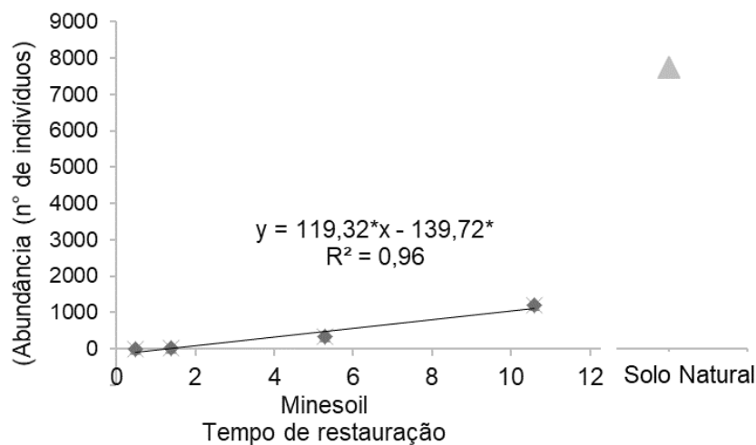
Figura 15 – Relação entre a abundância e o tempo de restauração dos minesoils ao longo de uma cronossequência de 10,6 anos.
