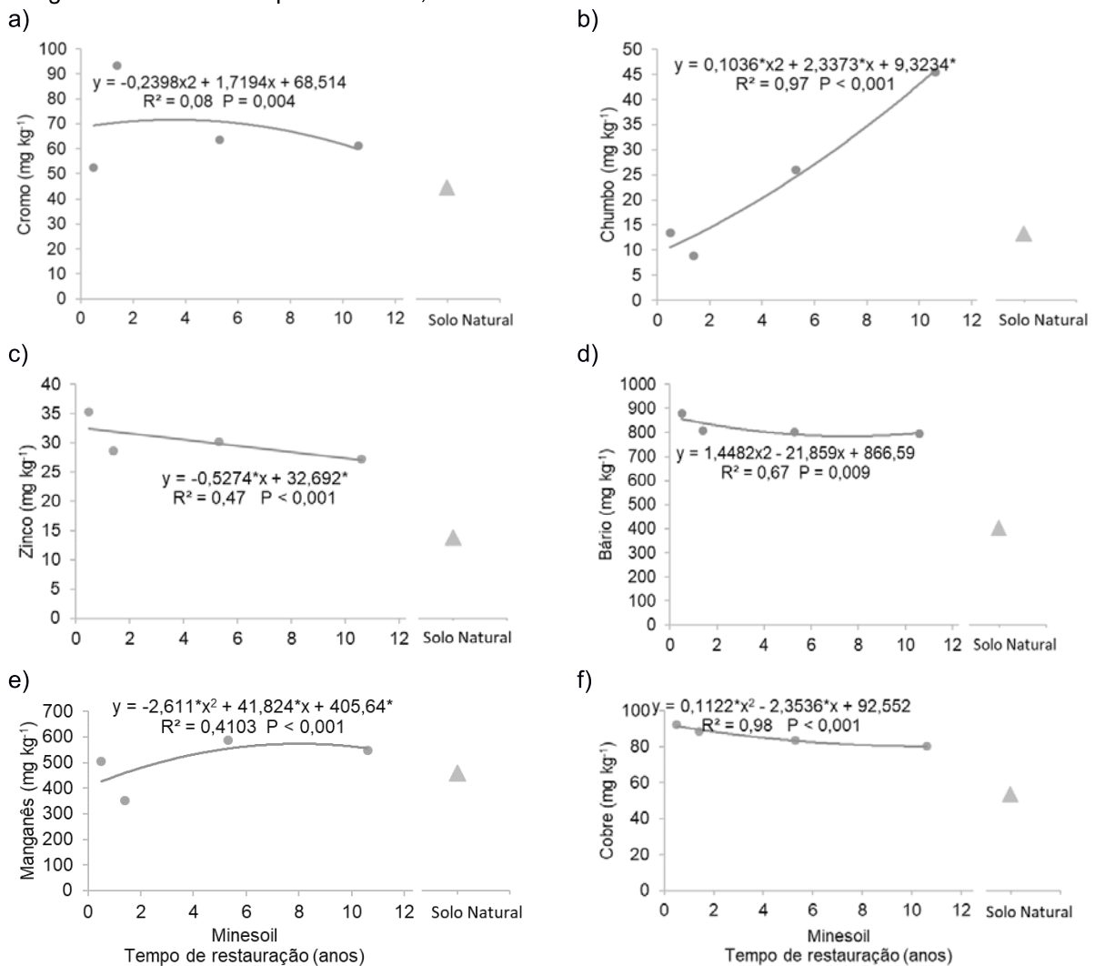
Figura 12 – Relação entre os teores de metais pesados e o tempo de restauração dos minesoils ao longo de uma cronosequência de 10,6 anos.
