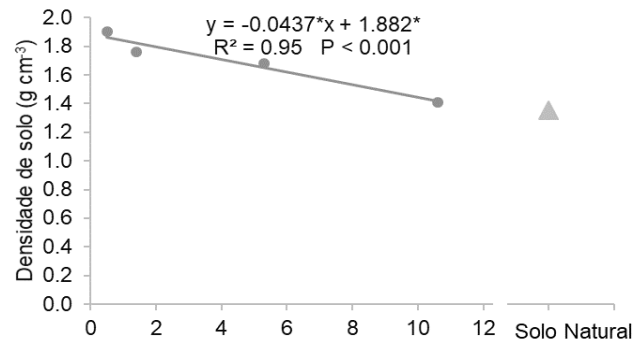
Figura 14 – Relação entre a densidade, macroporosidade e porosidade total e o tempo de restauração dos minesoils ao longo de uma cronossequência de 10,6 anos.
