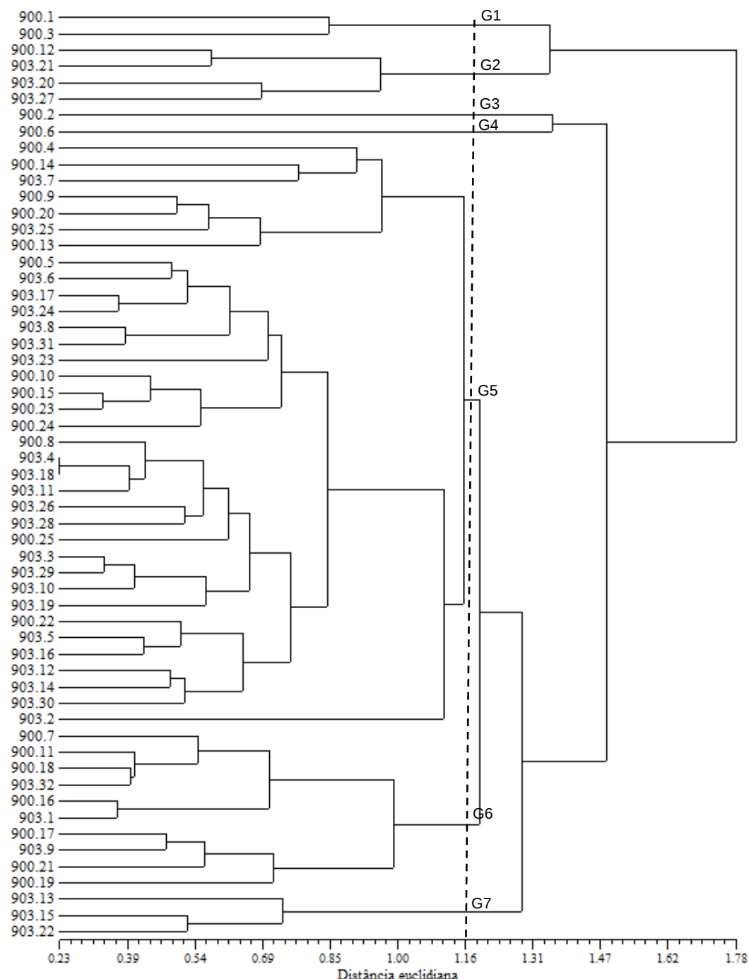
Figura 1. Dendrograma de dissimilaridade genética pelo método da média das distâncias para 57 genótipos de Macroptilium lathyroides baseado na distância Euclidiana para 22 caracteres morfoagronômicos. A linha tracejada indica a média das distâncias e o ponto de corte do dendrograma.
