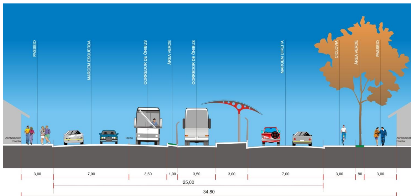
Figura A.3: Seção transversal padrão da Avenida Tronco/Porto Alegre (projeto).
