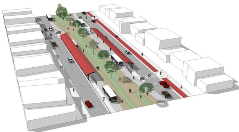
Figura A.4: Perspectiva do projeto de duplicação com estações na Avenida Tronco/Porto Alegre.
