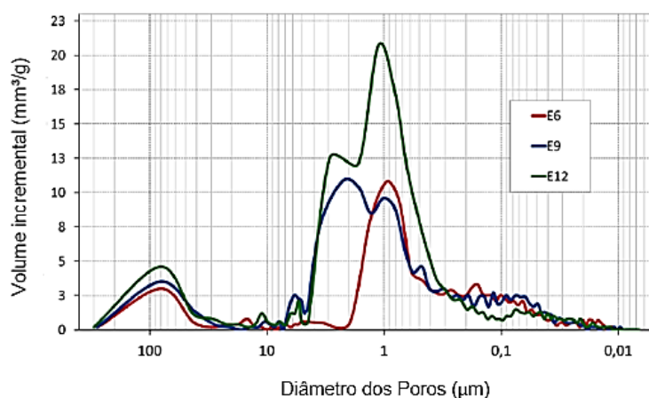
Figura 57 – Gráfico da distribuição de volume dos poros de três argamassas. Fonte: BAUER E SALOMÃO, 2017.
