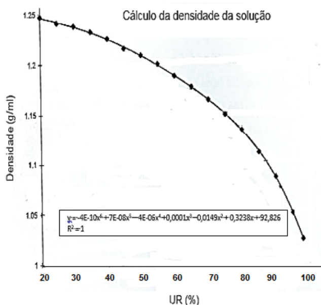
Figura 88 – Gráfico para cálculo da densidade da solução em função da UR. Fonte: Autor, Adaptado de ANTÓN, 2009.
