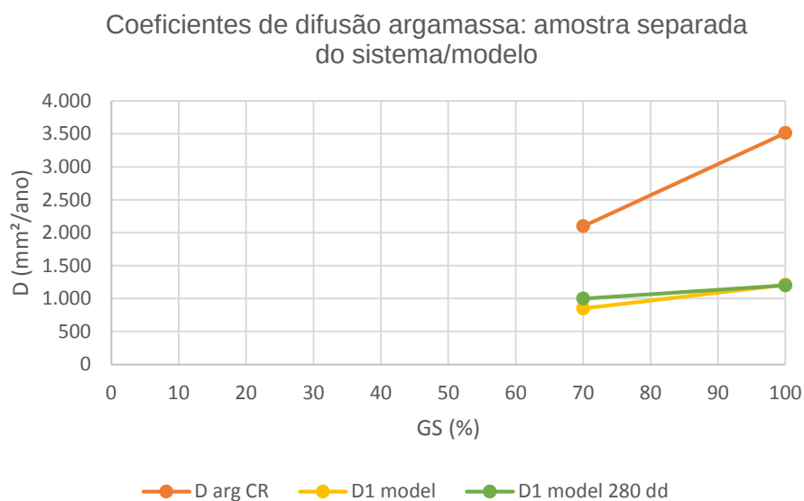
Figura 126 – Gráfico do coeficiente de difusão, em relação ao GS, para a argamassa na condição separada do sistema revestimento/concreto e no modelo (D1).
