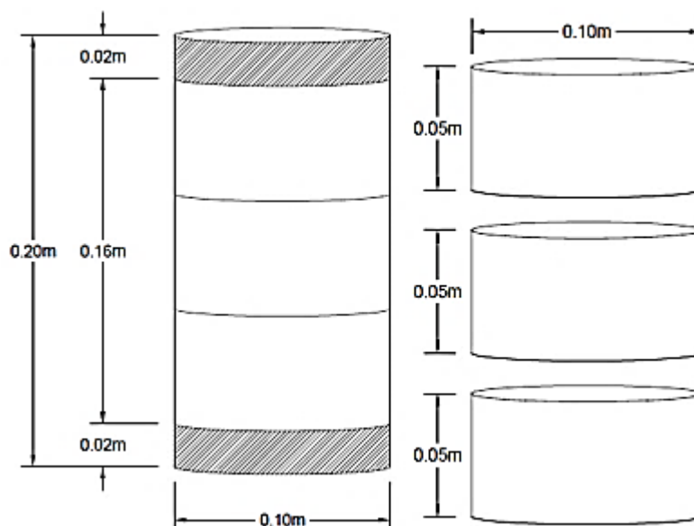
Figura 61 – Desenho esquemático dos cortes nos CPs de concreto. Fonte: Autor.
