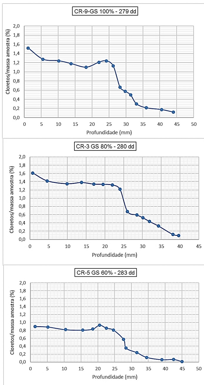
Figura 115 – Gráfico dos perfis de cloritos CPs tipo CR, para vários valores de GS, com 280 dias de difusão.
