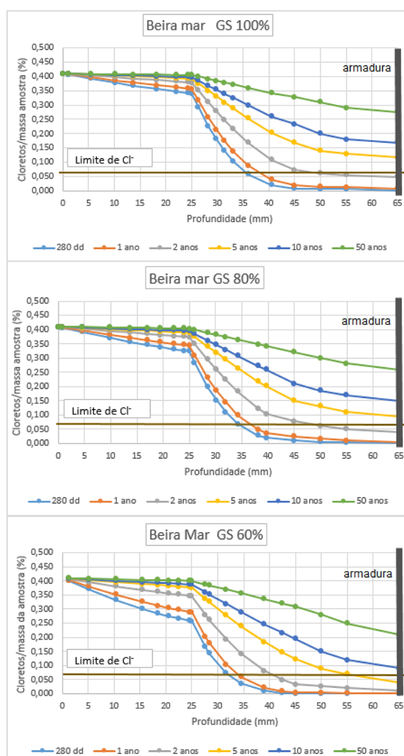
Figura 128 – Gráficos dos modelos de previsão da frente de ataque de cloretos em estruturas de concreto revestido com argamassa, considerando a variação do GS, localizadas à beira mar.
