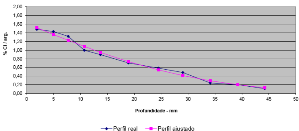
Figura 96 – Gráfico do perfil de penetração de cloretos ajustado. Fonte: Autor
