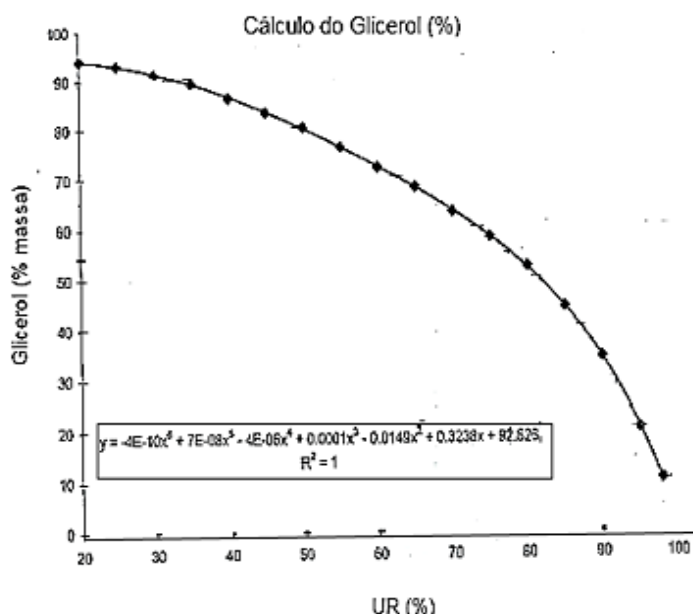
Figura 89 – Gráfico para cálculo do glicerol em função da UR. Fonte: Autor, Adaptado de ANTÓN, 2009.
