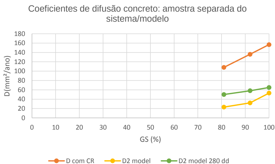
Figura 127 – Gráfico do coeficiente de difusão, em relação ao GS, para o concreto na condição separado do sistema revestimento/concreto e no modelo (D2).
