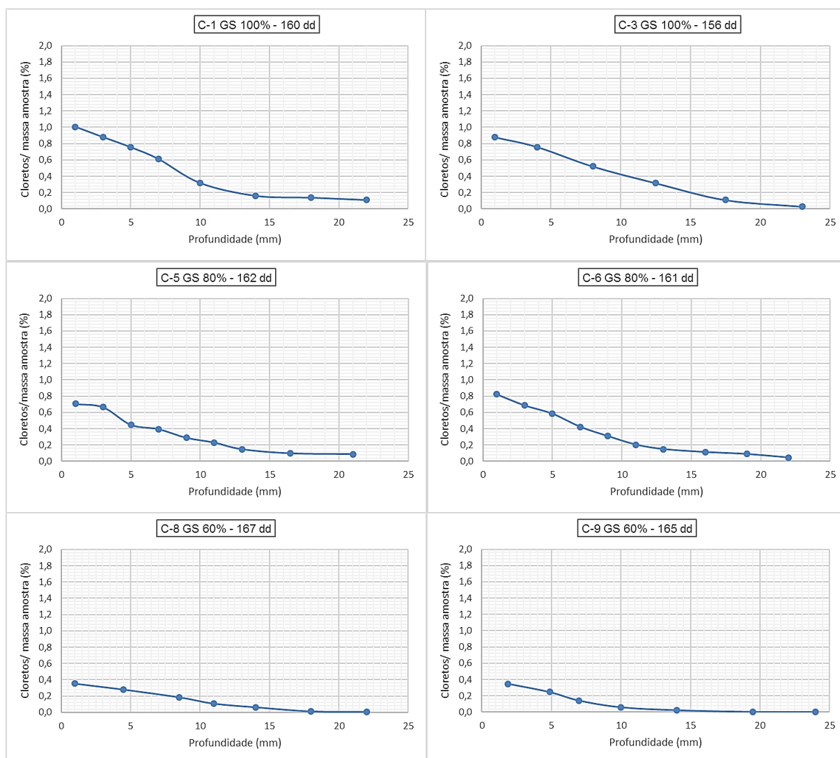
Figura 110 – Gráfico dos perfis de Cloretos CPs tipo C, para vários valores de GS. Fonte: Autor.
