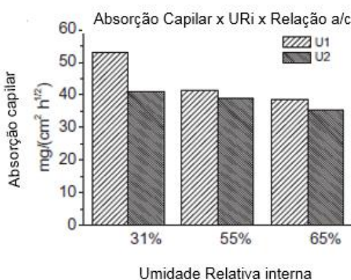
Figura 12 – Gráfico de coeficientes para absorção capilar em função da umidade relativa interna de concretos com relação a/c diferentes.
