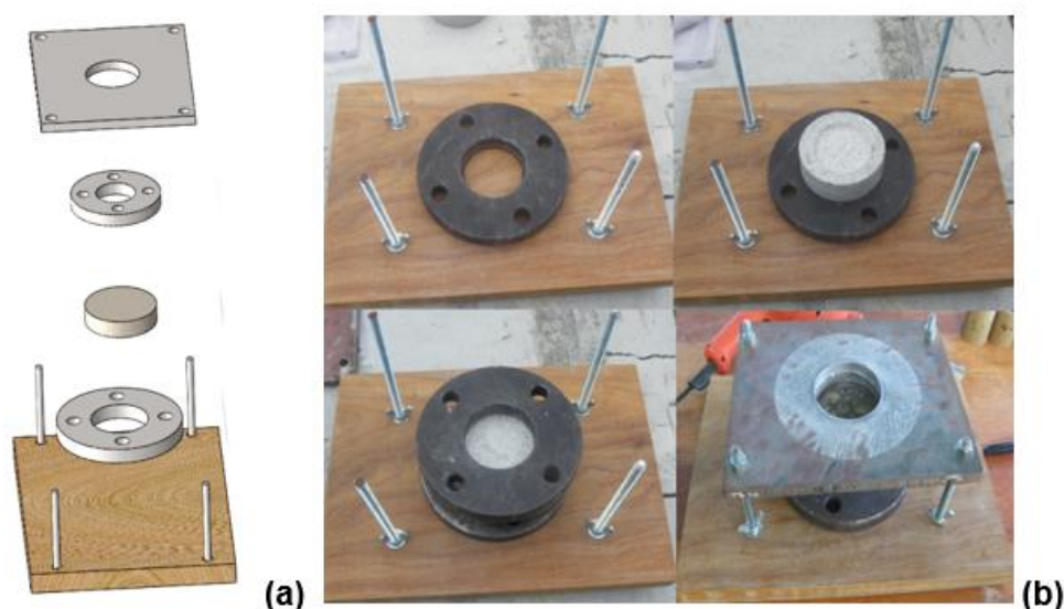
Figura 64 – Equipamento para extração: a) desenho esquemático; b) sequência de montagem do equipamento.
