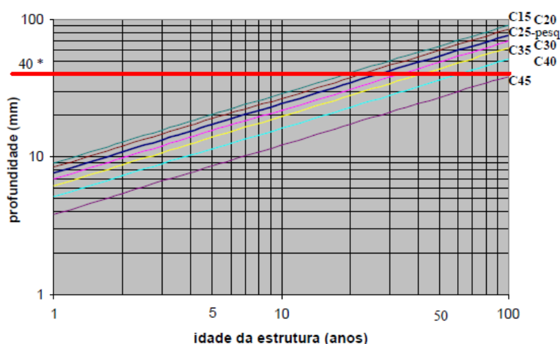
Figura 5 – Ábaco para estimar espessura de cobrimento de armaduras, em zona predominante de névoa. Considerando 40mm como cobrimento mínimo para ambiente marítimo pela norma NBR 6118 (ABNT, 2000).
