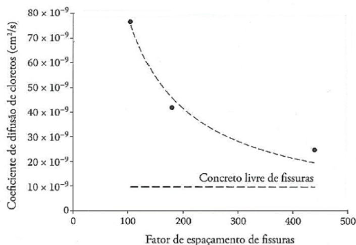
Figura 31 – Gráfico relacionando o coeficiente de difusão de cloretos e o fator de espaçamento de fissuras em concreto fissurado por ataque de congelamento-degelo.
