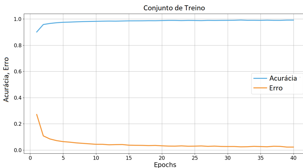
Figura 11 – Acurácia e erro na etapa de treino [O autor, 2021].
