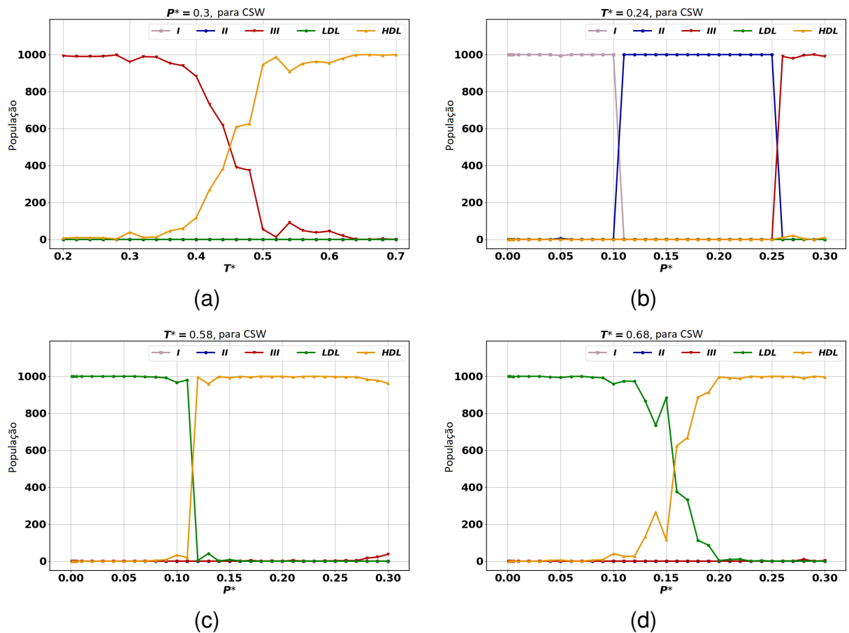
Figura 21 – População para água pura (a) em função da temperatura para pressão igual a 0.3, e como função da pressão para valores de temperatura igual a (b) 0.24, (c) 0.58 e (d) 0.68 [O autor, 2021].
