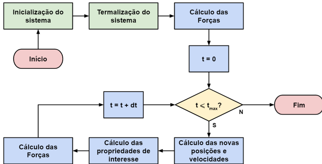
Figura 7 – Fluxograma do algoritmo típico de Dinâmica Molecular [O autor, 2021].
