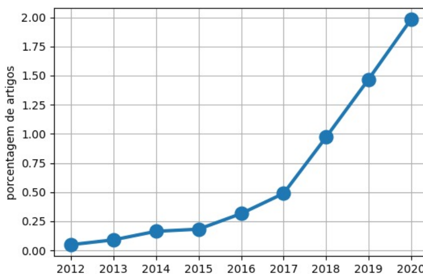
Figura 6 – Porcentagem de preprints publicados na seção de Física do repositório arXiv que contém o termo machine learning em seu resumo [O autor, 2021].
