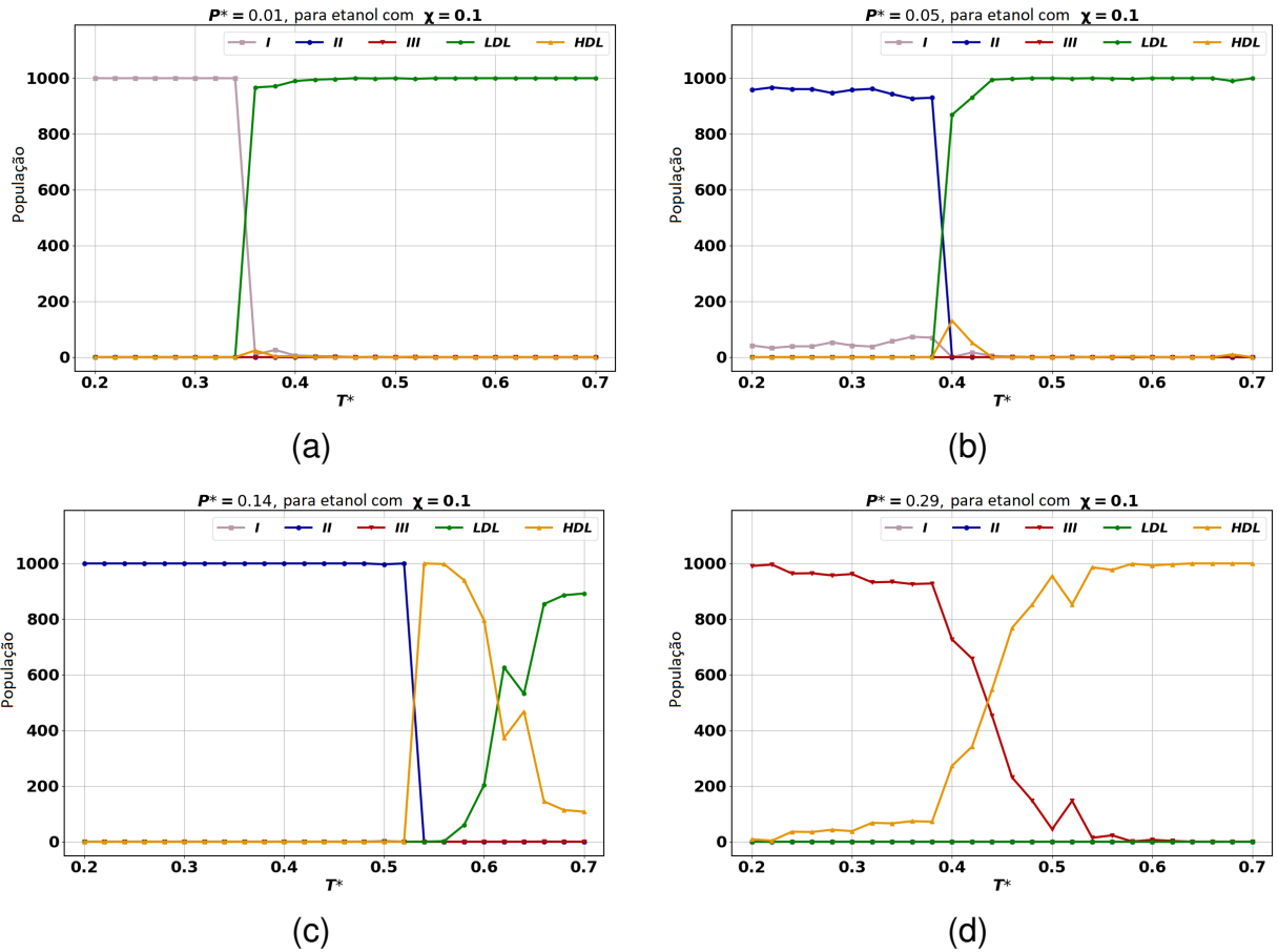
Figura 20 – Populações em função da temperatura para a mistura água-etanol com concentração igual a 0.1 e para valores de pressão igual a (a) 0.01, (b) 0.05, (c) 0.14 and (d) 0.29 [O autor, 2021].
